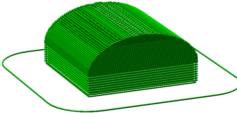
FIGURE 5.34 : Exemple avec une hauteur de couche variable.
