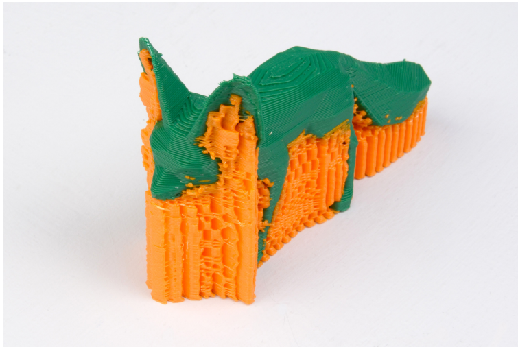
FIGURE 4.5 : Un exemple d'un objet imprimé avec un support.
