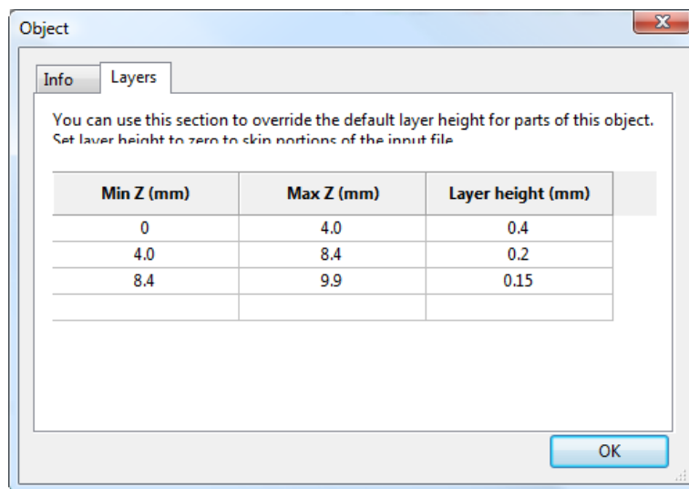
FIGURE 5.33 : Paramètres de Couche variable - Layers (Couches).
