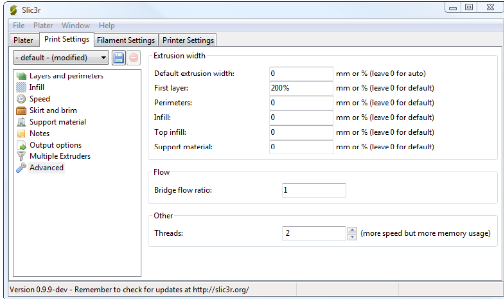
FIGURE 5.29 : Paramètres de largeur d'Extrusion.
