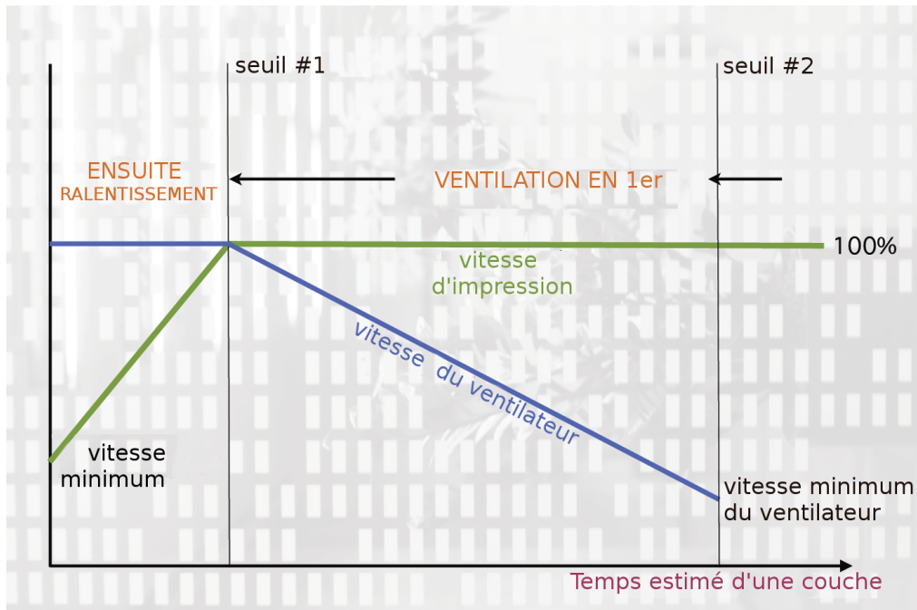
FIGURE 5.16 : Stratégie de refroidissement.
