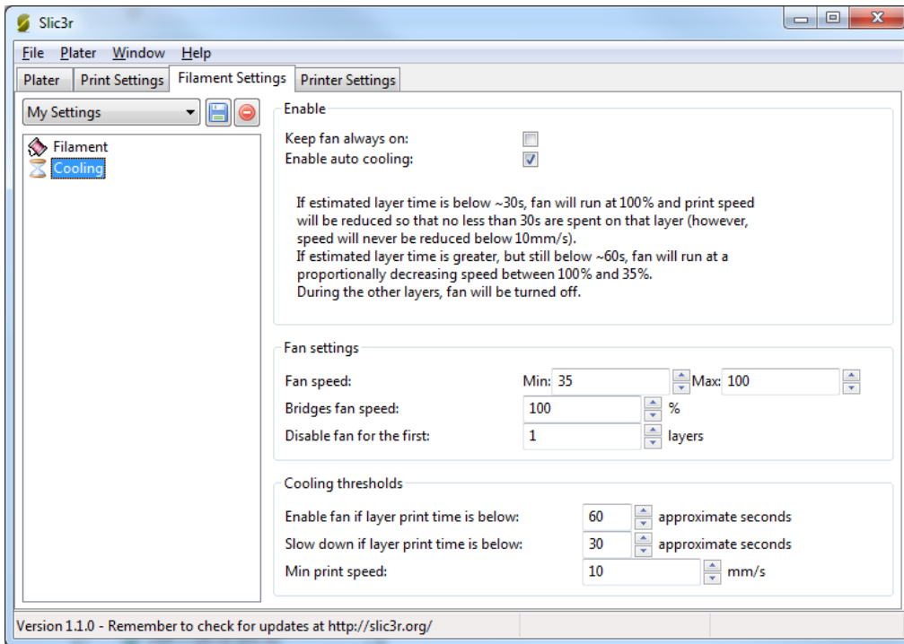
FIGURE 5.17 : Paramètres avancés de refroidissement
